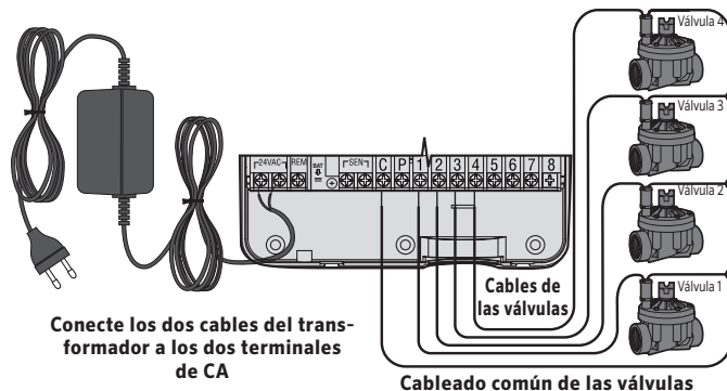
Cableado común de las válvulas
